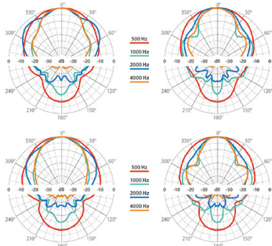
poziomy << wykres kołowy charakterystyki kierunkowej >> pionowy
