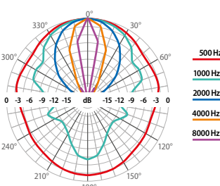
Wykres kołowy charakterystyki kierunkowej:
